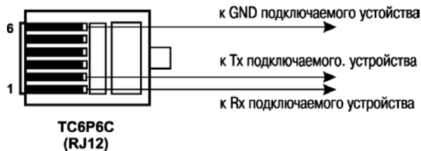
Рисунок В.2 - Схема распайки соединительного кабеля для подключения к порту RS-232 панели СМИ1
